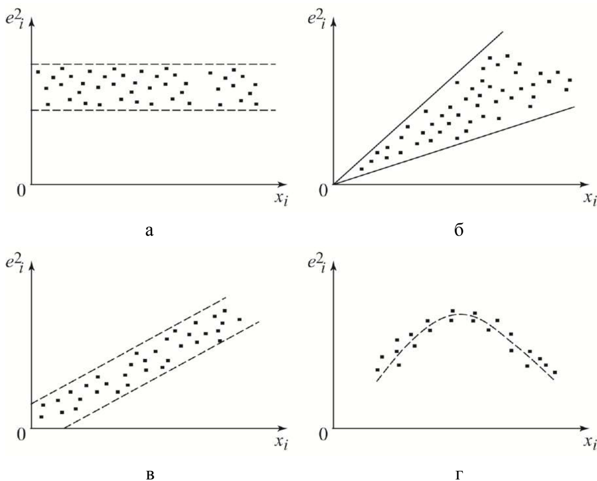
Рис. 23.2. Залежності \varepsilon_i^2 від x_i
