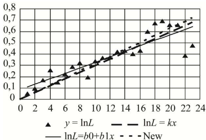
Рис. 25.6. Апроксимація часового тренду для \ln L
