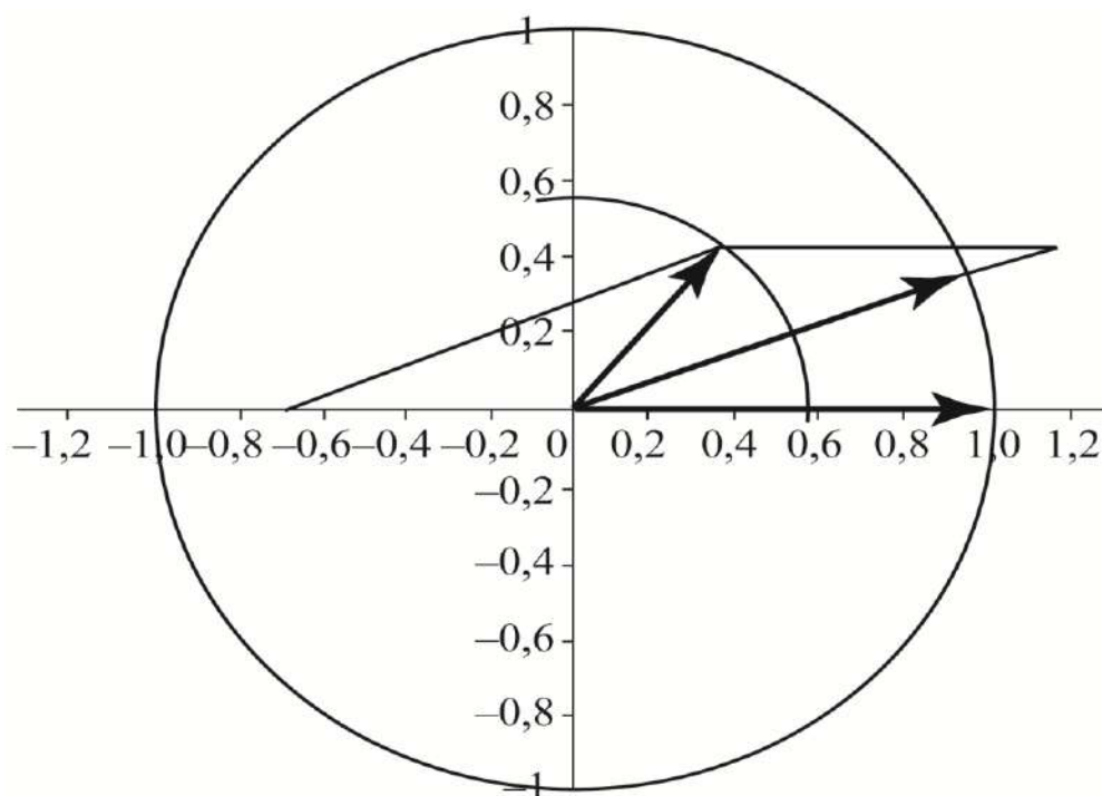
Рис. 25.2. Геометрична інтерпретація для першої моделі
