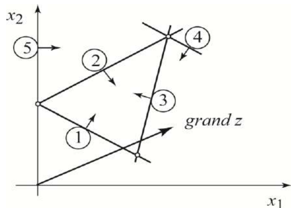
Рис. 3.11. Виродження плану
