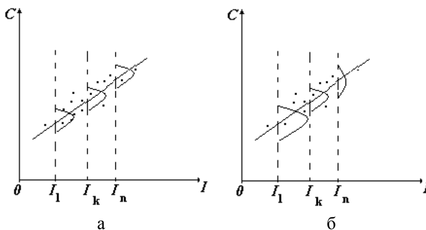
Рис. 23.1. а) гомоскедастичність залишків; б) гетероскедастичність залишків
