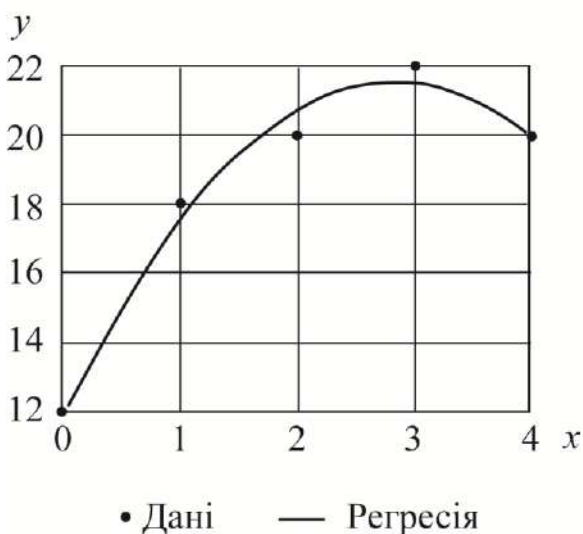
Рис.18.5. Квадратична залежність
