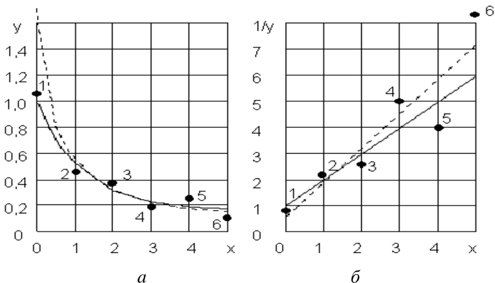
Рис. 23.3. Нелінійна залежність у вихідних змінних (а) і після функціональних перетворень (б),
