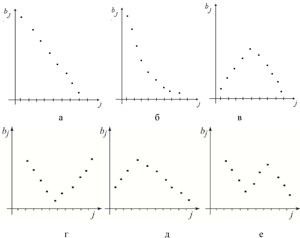
Рис. 28.1. Графічне зображення структури лага: а) лінійна, б) геометрична, в) перевернута V-подібна, г), д), е) поліноміальна
