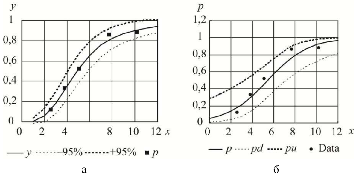
Рис. 26.7. Порівняння узагальненої лінійної моделі (а) з нелінійним регресійним аналізом (б)
