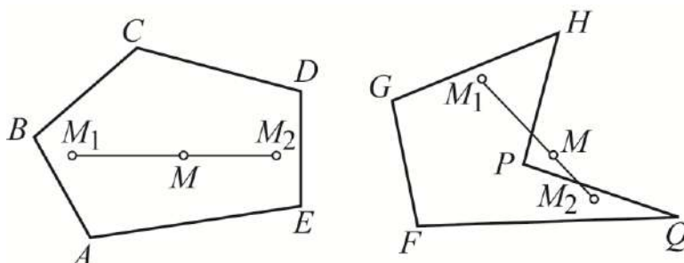
Рис. 3.16. Опукла ( ABCDE ) і неопукла ( FGHPQ ) множини
