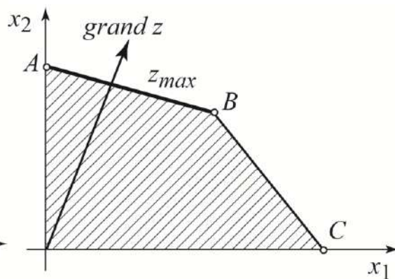
Рис. 3.7. Неєдиність оптимального розв'язку
