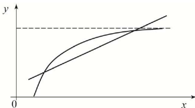
Рис. 24.4. Неправильна форма зв'язку
