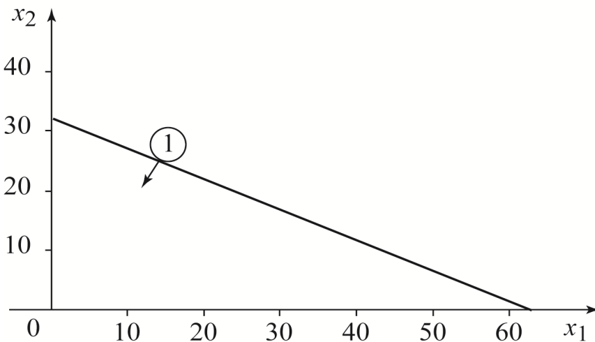
Рис. 3. 12. Область розв'язання 1-ї нерівності
