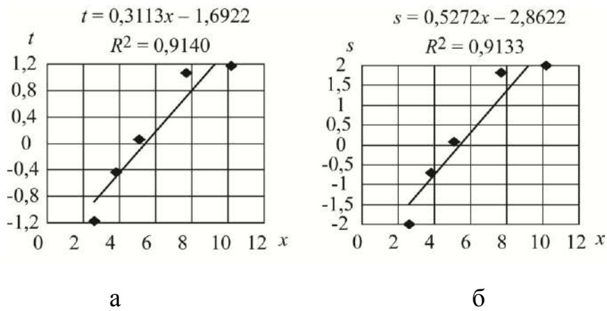
Рис. 26.4. Апроксимація залежності p(x) в функціональних змінних
