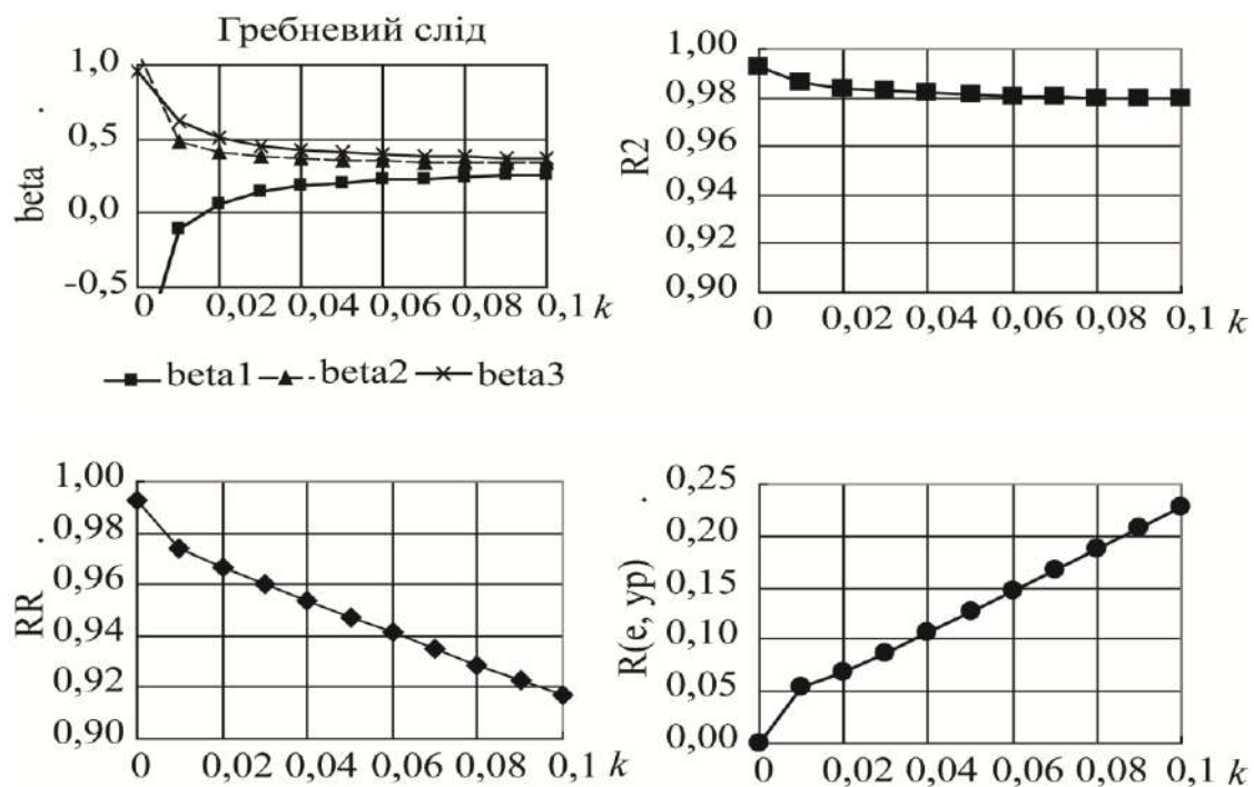
Рис. 22.2. Графіки залежності від ридж-параметра k
