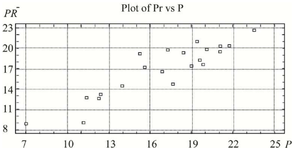
Рис. 27.1. Відповідність між P і P^R
