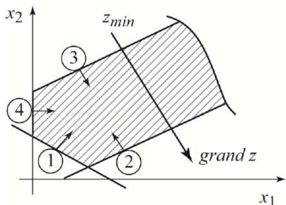
Рис. 3.8. Область планів відкрита, функція цілі – обмежена
