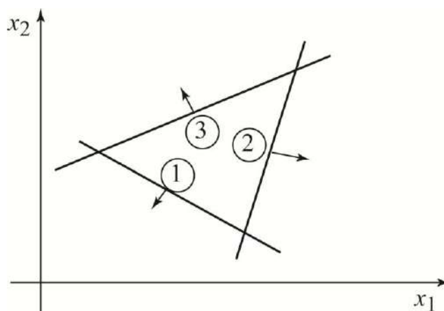
Рис. 3.5. Немає розв'язків
