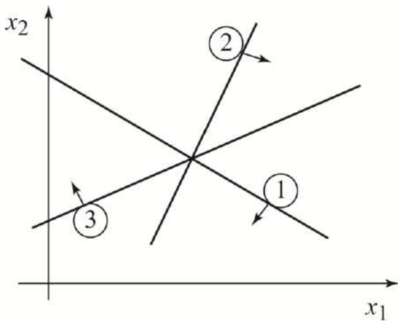
Рис. 3.9. Єдиний розв'язок
