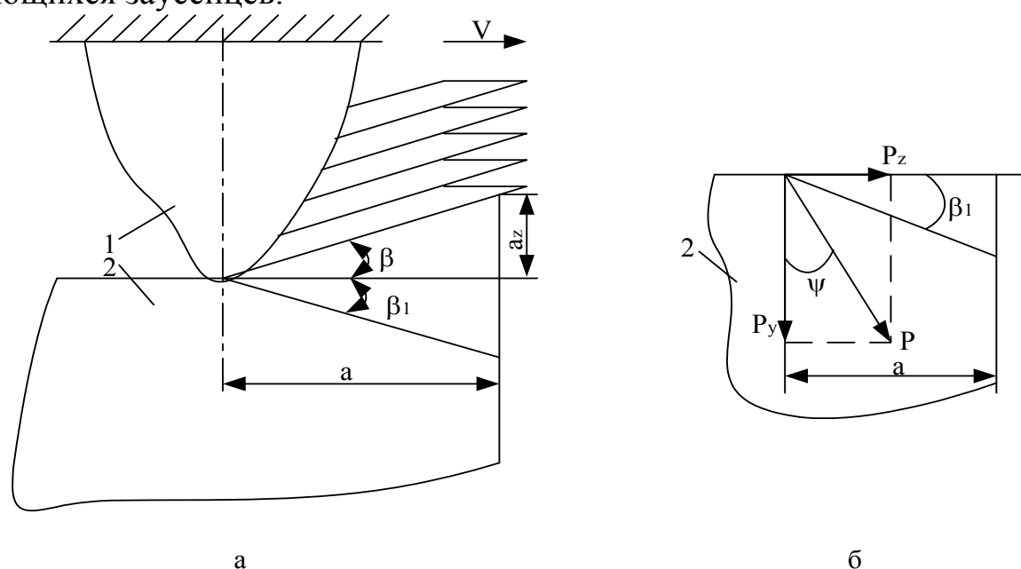
Рис. 1 Расчётная схема:
