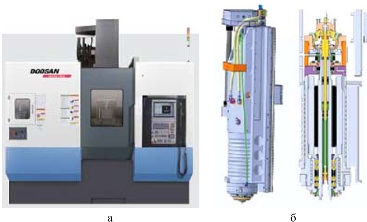
Рис. 6.2. Пятиосевой фрезерный обрабатывающий центр VC630/5AX (а) и мотор-шпиндель Built-in (б)
