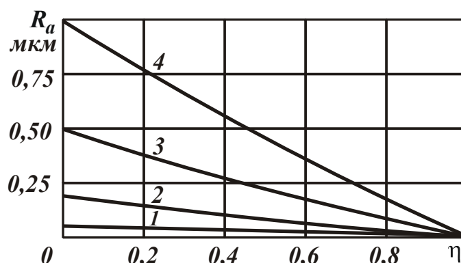
Рис. 4.13. Зависимость параметра шероховатости поверхности R_a от безразмерного коэффициента \eta для различных значений параметра R_{a0} : 1 – R_{a0} = 0,05 мкм; 2 – R_{a0} = 0,2 мкм; 3 – R_{a0} = 0,5 мкм; 4 – R_{a0} = 1 мкм
