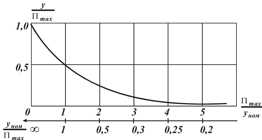
Рис. 3.10. Зависимость безразмерной величины y/\Pi_{max} от безразмерной величины \Pi_{max}/y
