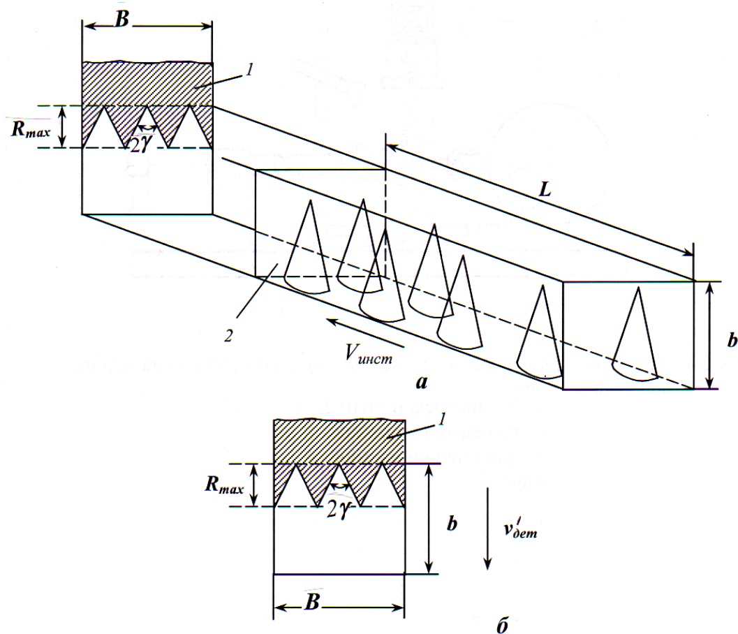
Рис. 4.1. Расчетная схема формирования шероховатости поверхности: 1 – обрабатываемая деталь; 2 – абразивный инструмент.
