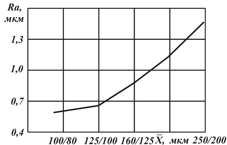
Рис. 4.15. Зависимость параметра шероховатости обработки R_a от зернистости круга \bar{X} : V_{дет} = 0,6 м/мин; V_{кр} = 28 м/с
