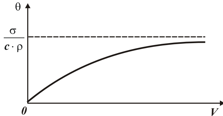
Рис. 4.21. Примерная зависимость температуры резания \theta от скорости резания V
