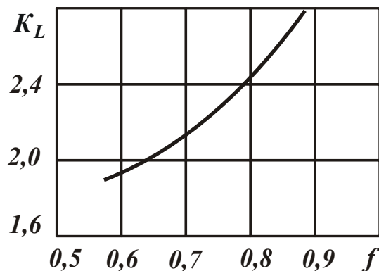
Рис. 1.21. Зависимость K_L от f : обрабатываемый материал – сталь 30; t=4 мм; S = 0,125 \dots 0,78 мм/об.; V = 35 \dots 270 м/мин
