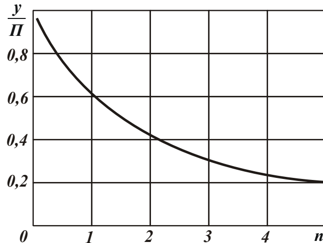
Рис. 2.8. Зависимость отношения y/\Pi от количества проходов n
