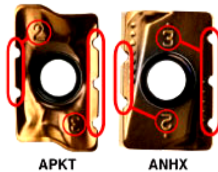
Рис. 6.58. Пластины с геометрией SM
