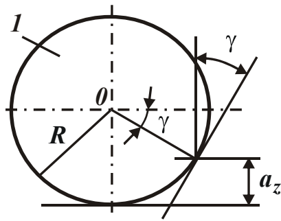
Рис. 3.23. Расчетная схема процесса микрорезания единичным зерном (1)
