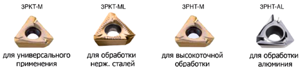
Рис. 6.46. Виды стружколомающей геометрии пластин серии АРКТ
