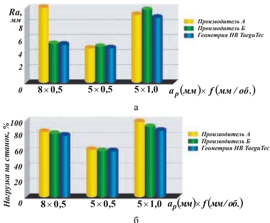
Рис. 6.25. Результаты по чистоте поверхности Ra (а) и по усилию резания (б)
