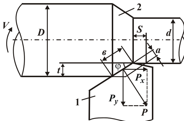
Рис. 1.2. Расчетная схема продольного точения: 1 – резец; 2 – деталь
