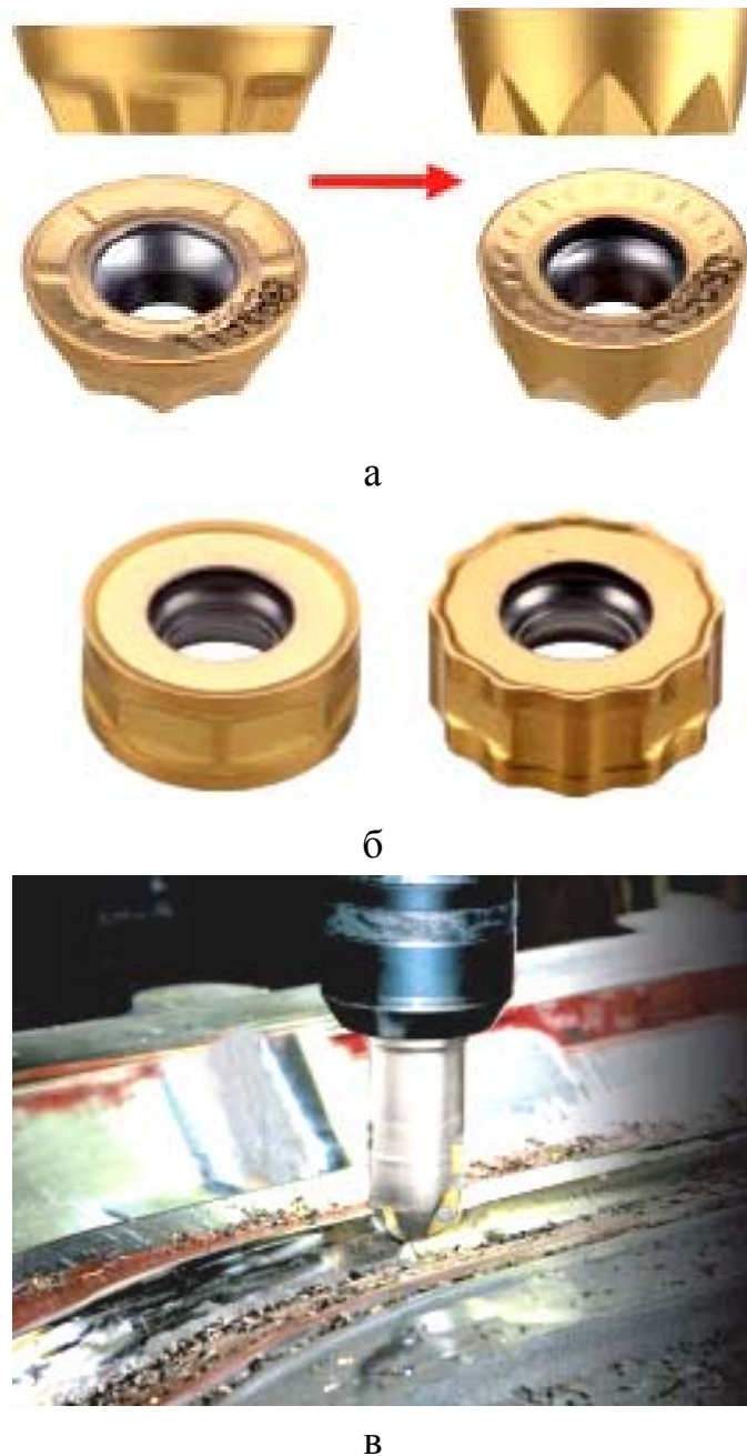
Рис. 6.50. Модернизация пластины RYMX (а), двухсторонняя пластина RNHU с 16-ю режущими кромками (б) и сферическая фреза TRIOBALL (в)
