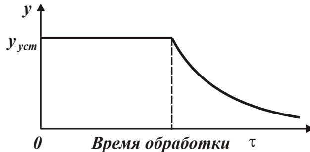
Рис. 2.14. Зависимость величины упругого перемещения y от времени обработки \tau (цикл шлифования, включающий этап черного шлифования и выхаживания)
