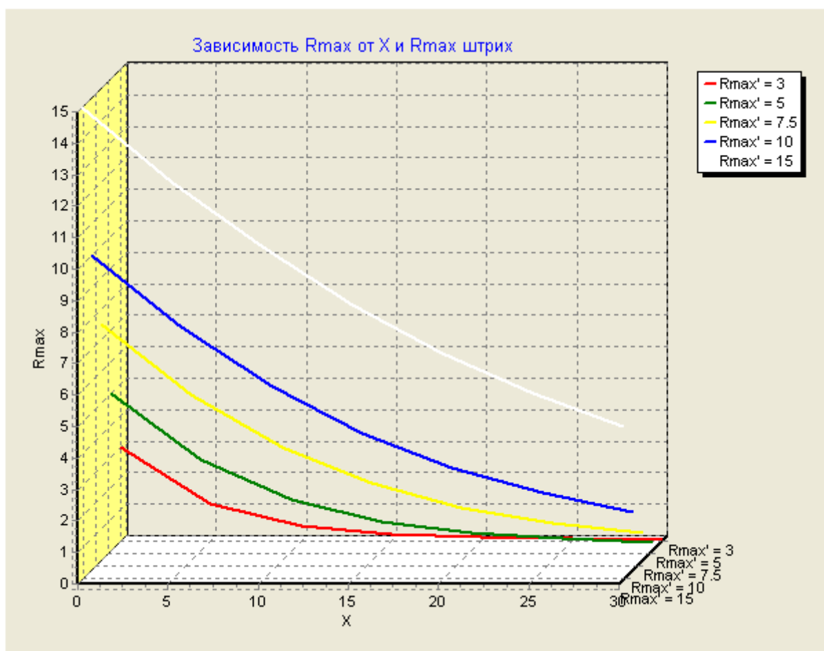
Рис. 4.18. Зависимость R_{max} от x для разных значений \bar{R}_{max} , установленная на основе решения уравнения (4.76)
