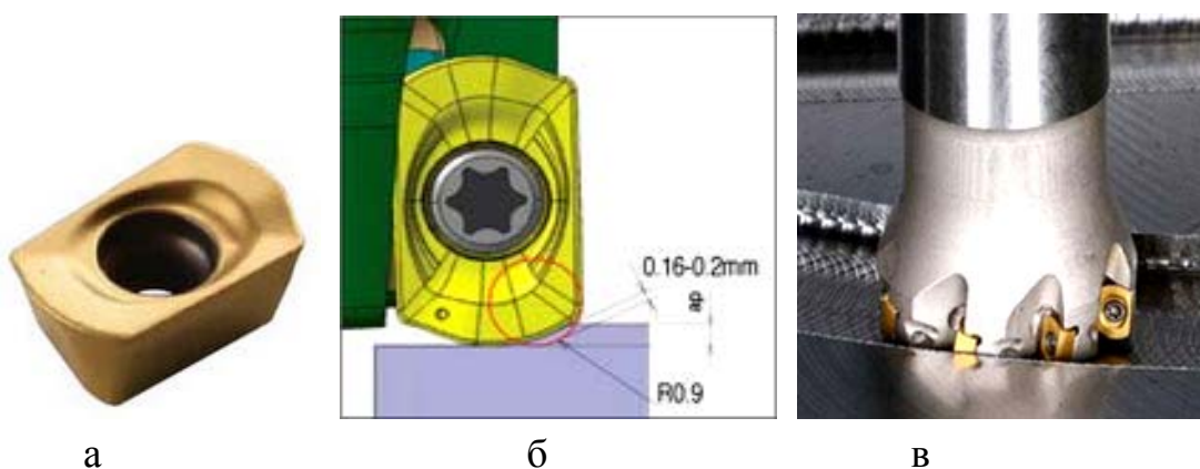
Рис. 6.72. Пластина небольшого габарита AXMT 0602R-HF (а) и программируемый радиус при ее вершине (б), фреза ChaseMill Mini (в)
