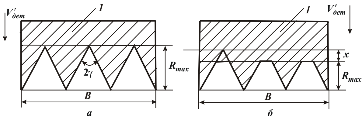
Рис. 4.16. Схемы образования шероховатости поверхности без учета (а) и с учетом (б) образования площадок износа на режущих зернах круга:
