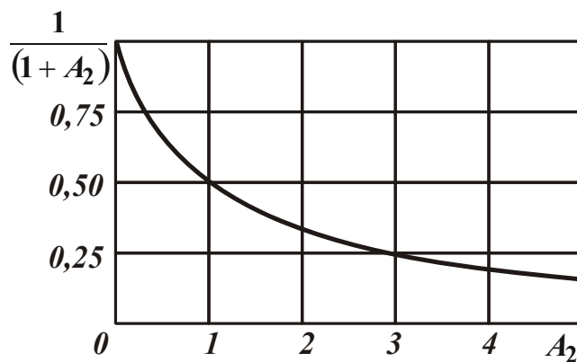
Рис. 2.4. Зависимость коэффициента 1/(1 + A_2) от A_2
