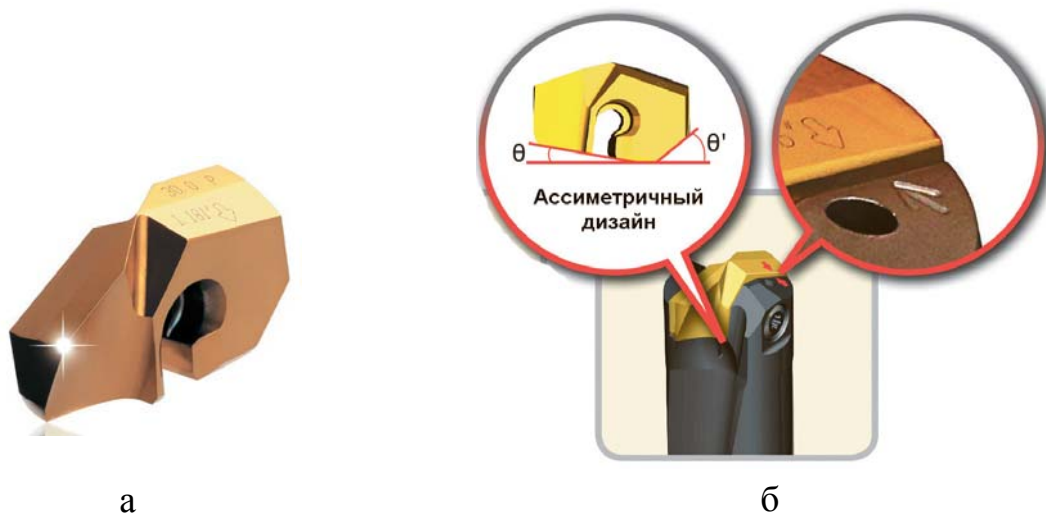
Рис. 6.106. Быстросменная твердосплавная головка (а) и ассиметричный дизайн посадочного места коронки SPADERUSH (б)
