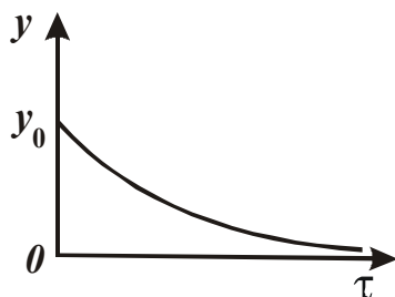
Рис. 3.5. Зависимость величины упругого перемещения y от времени обработки \tau для случая Q_0 = 0 ( V_0 = 0 )
