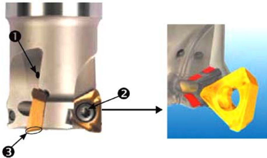
Рис. 6.47. Корпус фрезы серии MILLRUSH
