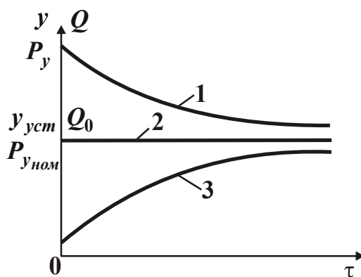
Рис. 5.9. Примерные зависимости параметров Q_{тек} , y и P_y от \tau
