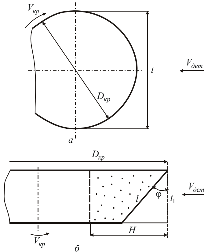
Рис. 5.2. Расчетные схемы плоского шлифования торцом круга
