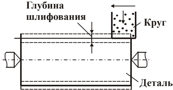
Рис. 2.9. Схема круглого наружного продольного шлифования
