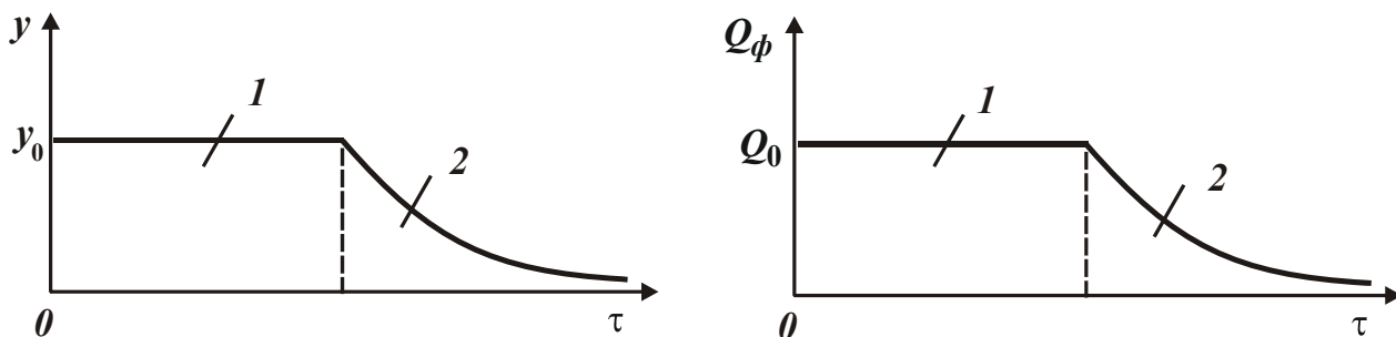
Рис. 3.6. Зависимости величины упругого перемещения y (а) и фактической производительности обработки Q_{\phi} (б) от времени обработки \tau :
