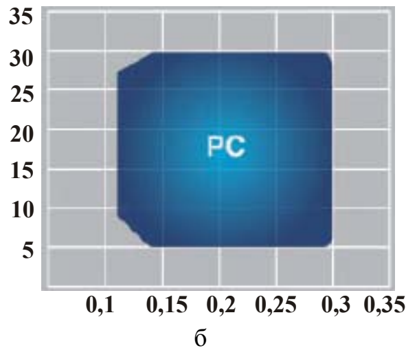
Рис. 6.23. Стружколом со стружколомающей геометрией РС (а) и область его применения (б)
