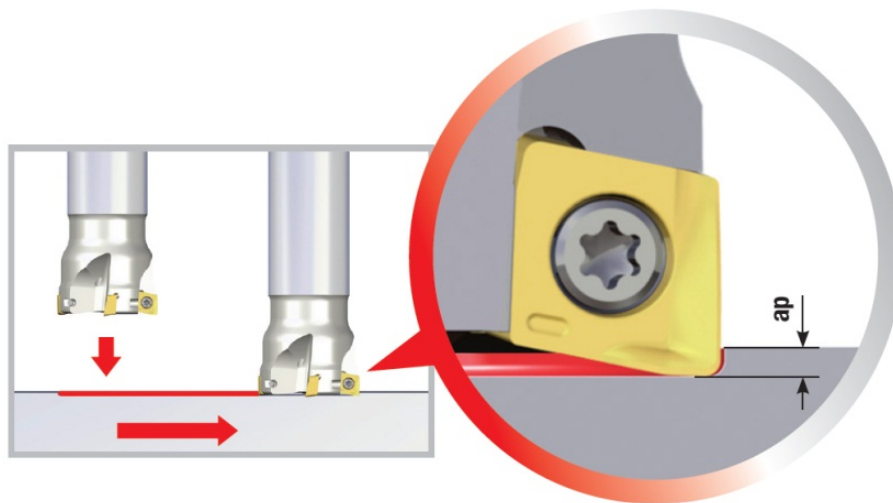
Рис. 6.91. Врезание торцом фрезы в металл по циклу сверления
