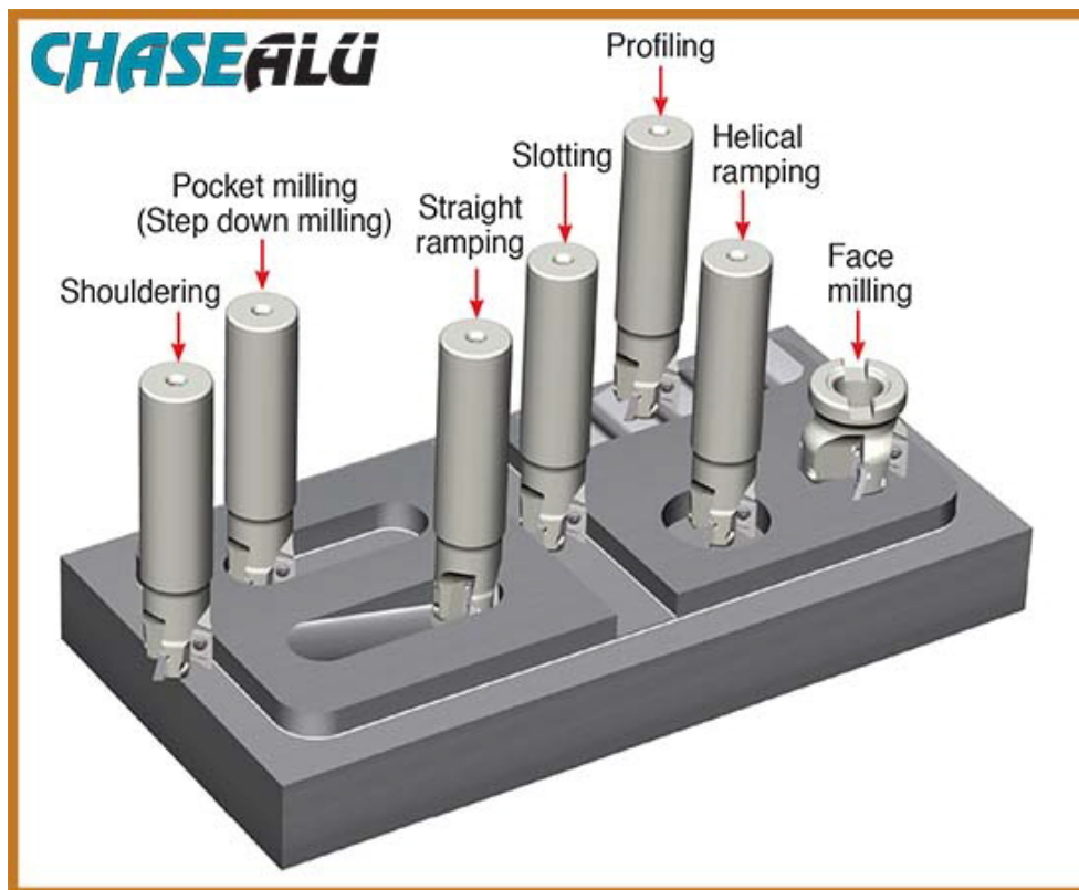
Рис. 6.80. Применение инструментов серии ChaseAlu при фрезеровании различных поверхностей
