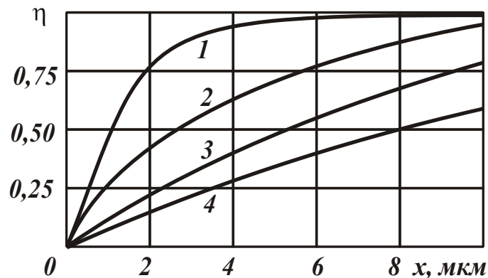
Рис. 4.12. Зависимость безразмерного коэффициента \eta от величины x для различных значений параметра H_0 : 1 – H_0 = 2 мкм; 2 – H_0 = 6 мкм; 3 – H_0 = 10 мкм; 4 – H_0 = 15 мкм
