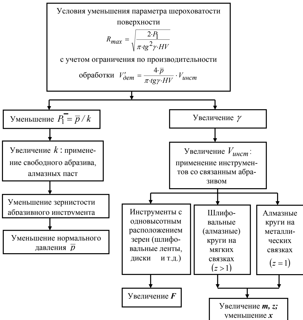
Рис. 4.4. Структурная схема условий уменьшения параметра шероховатости обработки R_{max}
