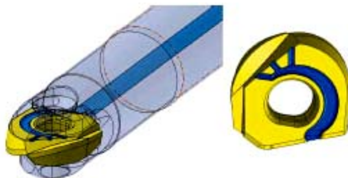
Рис. 6.53. Система подачи СОЖ через пластину
