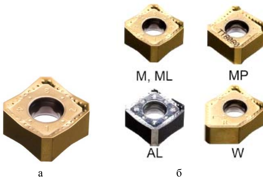
Рис. 6.65. Квадратная твердосплавная пластина серии SNGX 1205 (а) и геометрические конфигурации передней режущей поверхности пластин (б)
