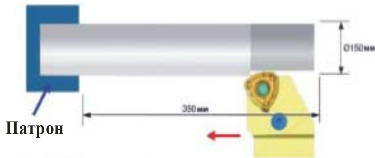
Рис. 6.28. Область применения пластин с геометрией HF (а) и эскиз обработки детали (б)
