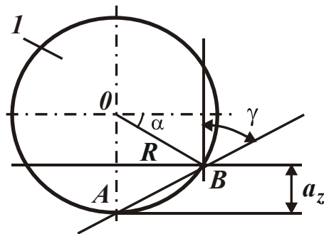
Рис. 3.26. Расчетная схема процесса микрорезания единичным зерном (1)
