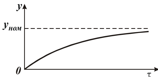
Рис. 3.2. Зависимость величины упругого перемещения y от времени обработки \tau
