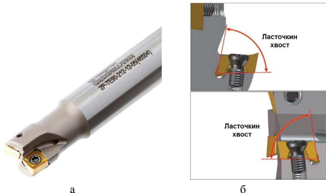
Рис. 6.89. Фреза серии CHASEMILL POWER (а) и посадочное место для пластины в виде "ласточкиного хвоста" (б)
