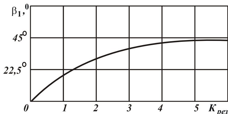
Рис. 1.29. Зависимость угла \beta_1 от K_{рез}
