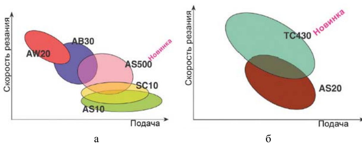
Рис. 6.19. Область эффективного применения керамических сплавов при обработке чугуна (а) и область эффективного применения керамических сплавов при обработке жаропрочных материалов (б)
