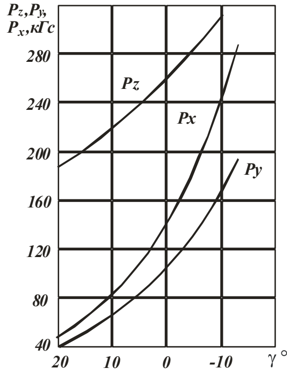
Рис. 1.12. Влияние переднего угла на силы P_z , P_y , P_x при точении: обрабатываемый материал – сталь 40; \varphi=60^\circ ; t=4 мм; S=0,285 мм/об.; V=40 м/мин [6]
