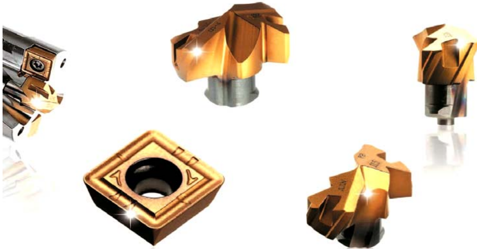
Рис. 6.96. Режущие пластины и коронки для обработки отверстий
