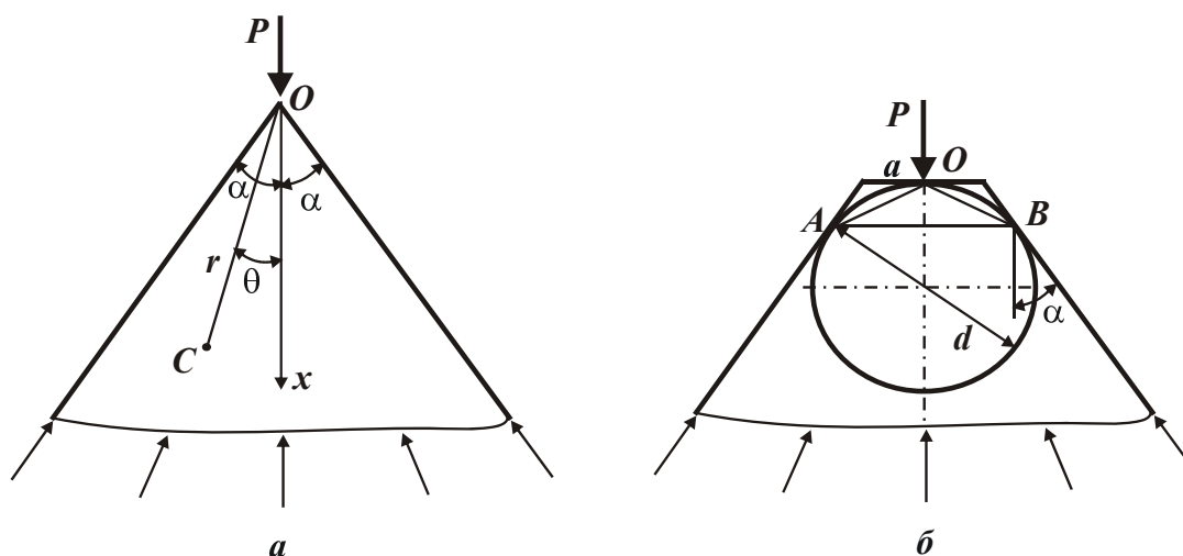
Рис. 1.26. Расчетные схемы напряжений в клине при действии радиальной силы
