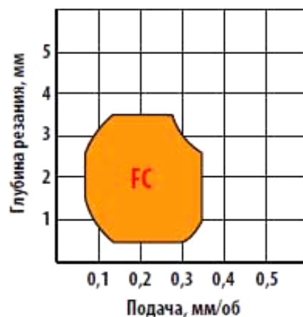
Рис. 6.6. Режущие пластины со стружколомающей геометрией РС и область их применения (а) и режущие пластины со стружколомающей геометрией FC и область их применения (б)
