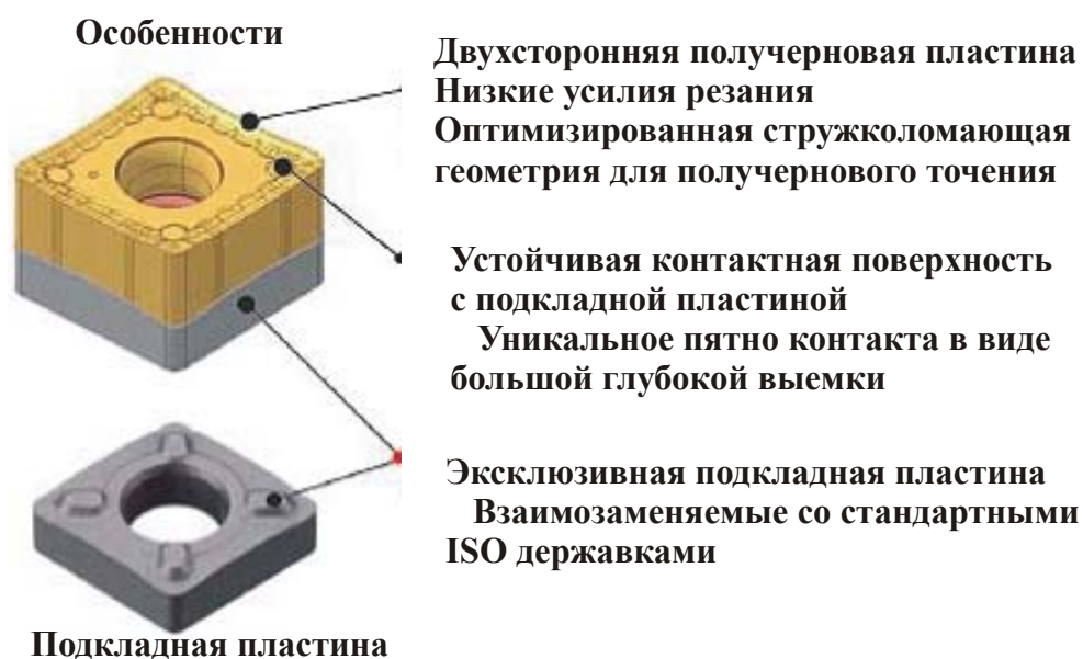
Рис. 6.24. Особенности пластин со стружколомающей геометрией НВ
