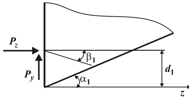
Рис. 1.28. Расчетная схема положения плоскости скола инструмента
