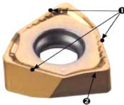
Рис. 6.48. Фрезы серии MILL2RUSH (а) и двухсторонняя пластина 6NGU (б)
