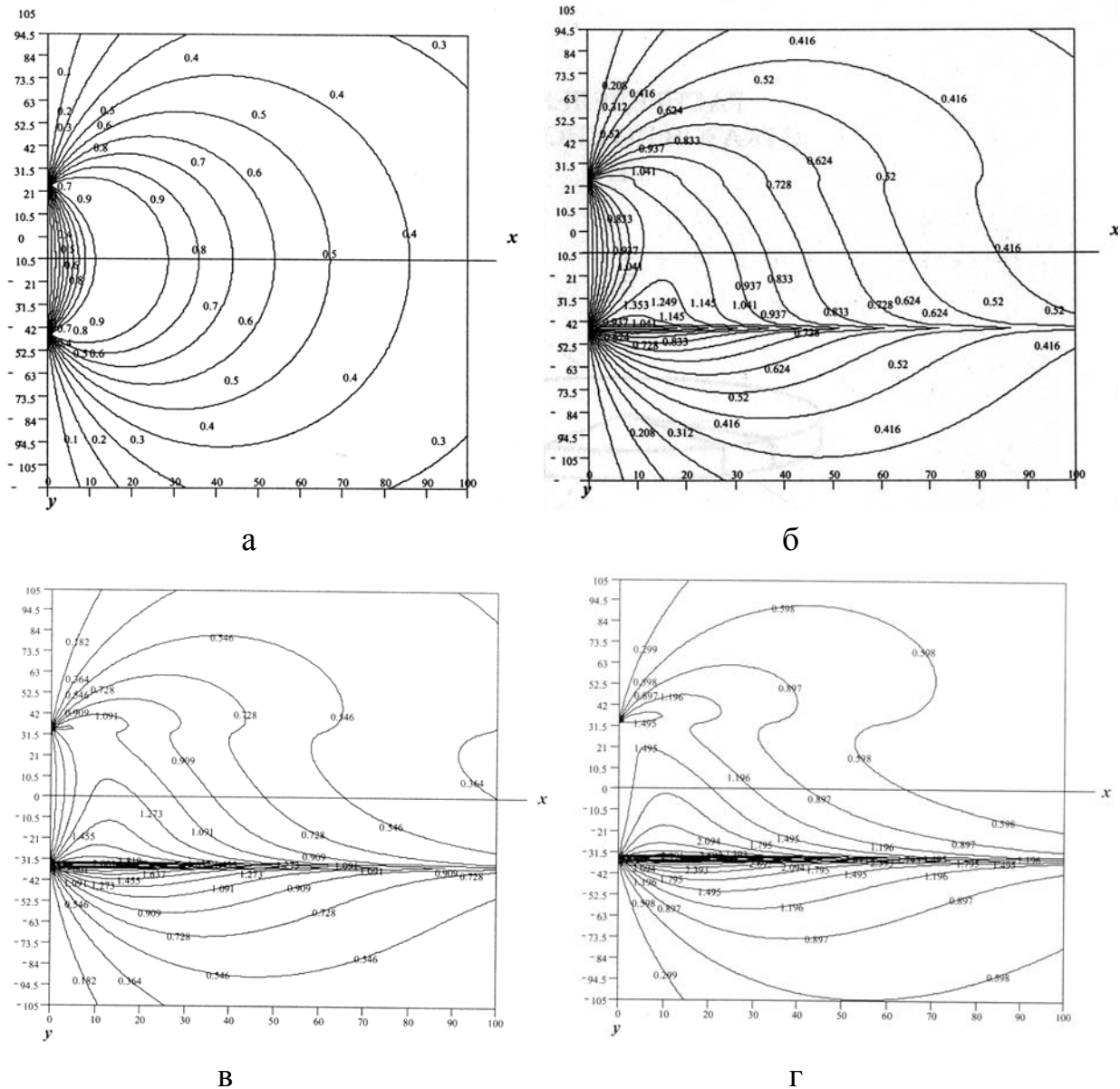
Рис. 1.25. Положения линий одинаковых значений \tau/q при f=0 (а), f=0,1 (б); f=0,4 (в); f=0,6 (г)
