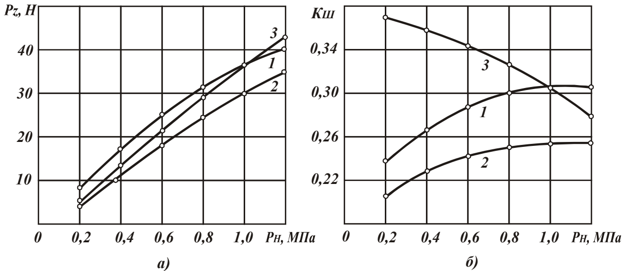
Рис. 1.14. Влияние нормального давления на тангенциальную составляющую силы резания и коэффициент шлифования: круг 12A2-45 0 АС6 100/80 М1-01 4, V = 20 м/с, обрабатываемый материал: 1 – Т15К6 – сталь 45-АЭШ, 2 – ТН-20 – сталь 45 – АЭШ, 3 – ТН-20-сталь 45 – АШ (по данным Малыхина В. В. [48])
