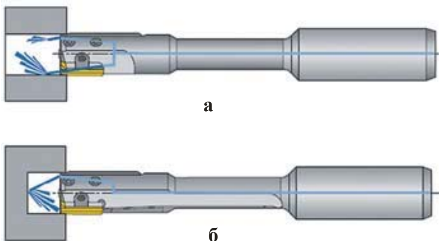
Рис. 6.108. Работа системы внутреннего подвода СОЖ в развертках ТВ-TEAM при получении сквозных (а) и глухих (б) отверстий
