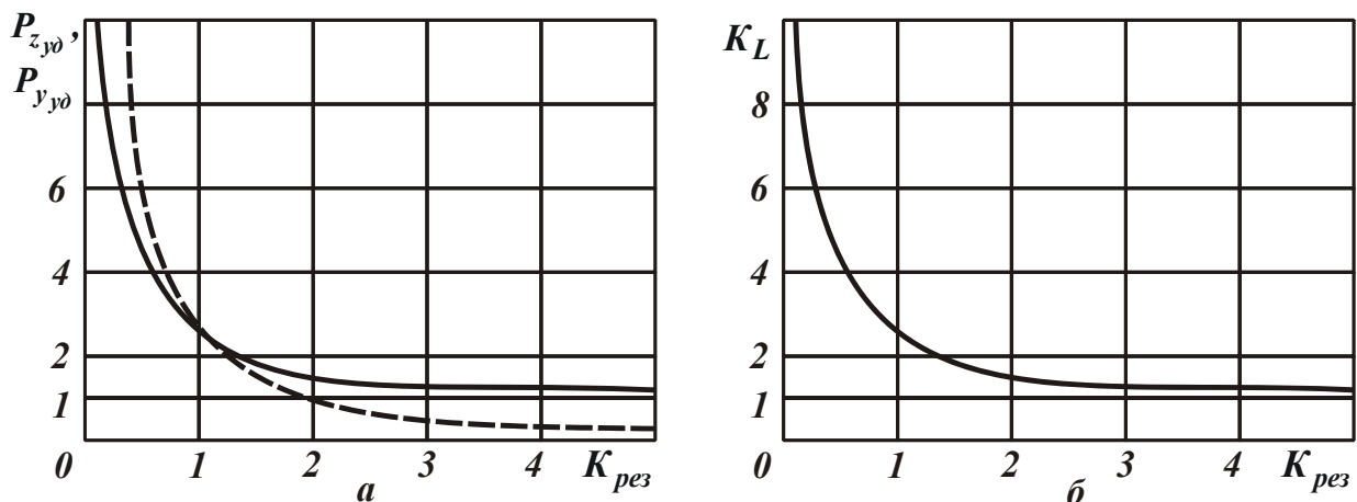
Рис. 1.8. Зависимости P_{z_{y\delta}} (сплошная линия) и P_{y_{y\delta}} (пунктирная линия) от K_{рез} (а) и K_L от K_{рез} (б).
