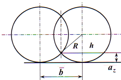
Рис. 5.3. Расчетная схема формирования микронеровностей на обрабатываемой поверхности
