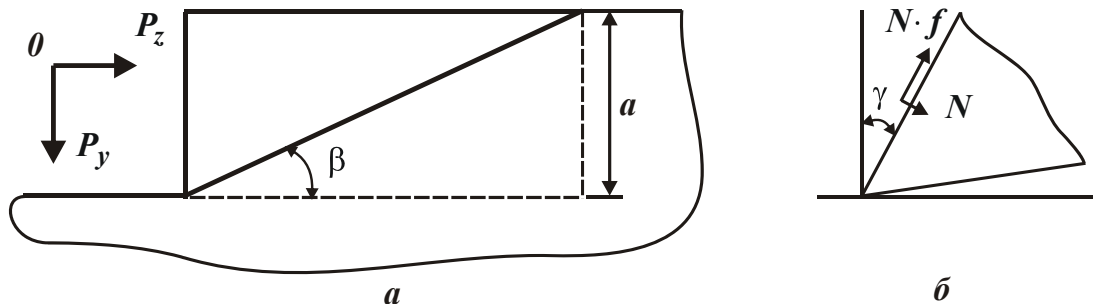
Рис. 1.4. Расчетная схема параметров стружкообразования при резании (а) и схема сил, действующих на передней поверхности инструмента (б)
