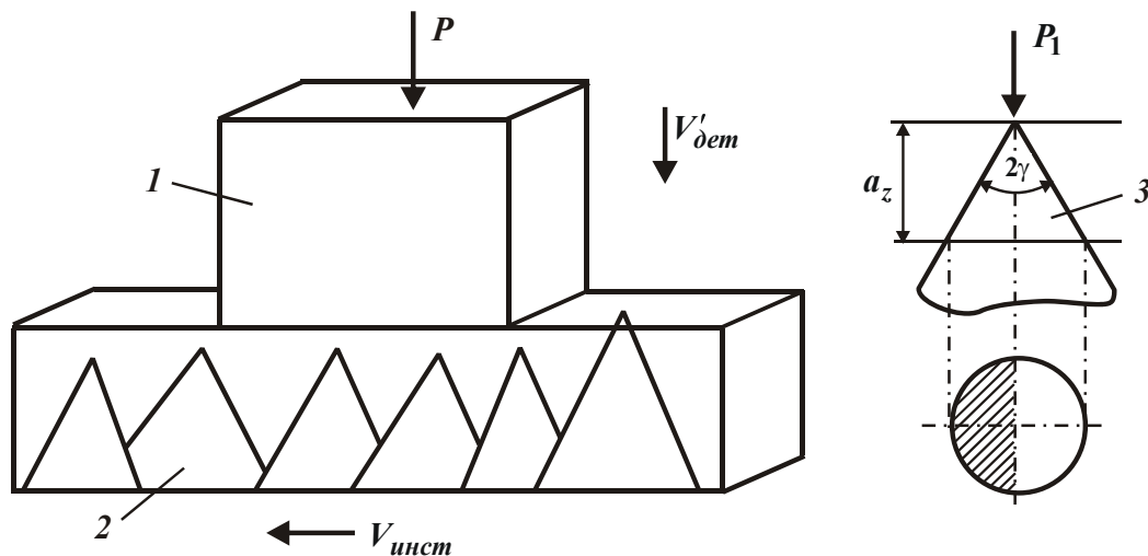
Рис. 4.2. Расчетная схема упругой схемы обработки с постоянным радиальным усилием P :
