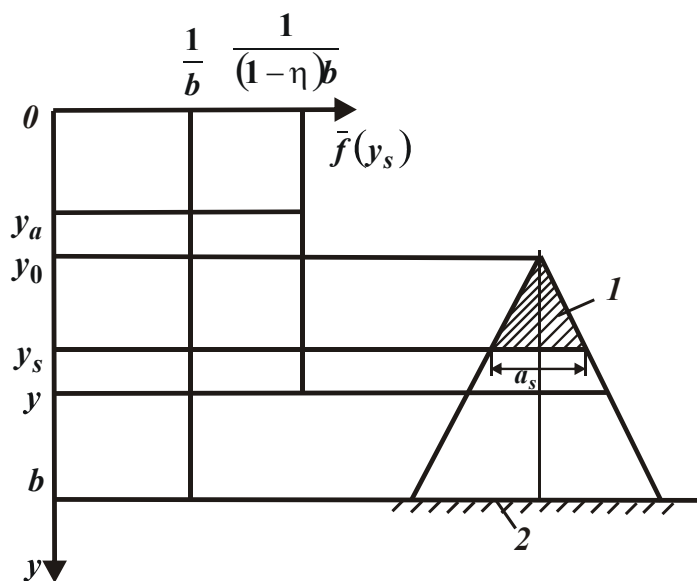
Рис. 4.8. Расчетная схема параметров изношенной части зерна 1 – изношенная часть зерна; 2 – уровень связки круга
