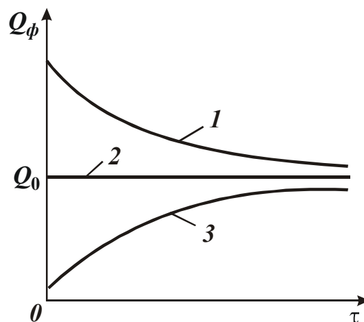
Рис. 3.3. Зависимость фактической производительности обработки Q_{\phi} от времени обработки \tau : 1 – y_0 > y_{ном} ; 2 – y_0 = y_{ном} ; 3 – y_0 < y_{ном}
