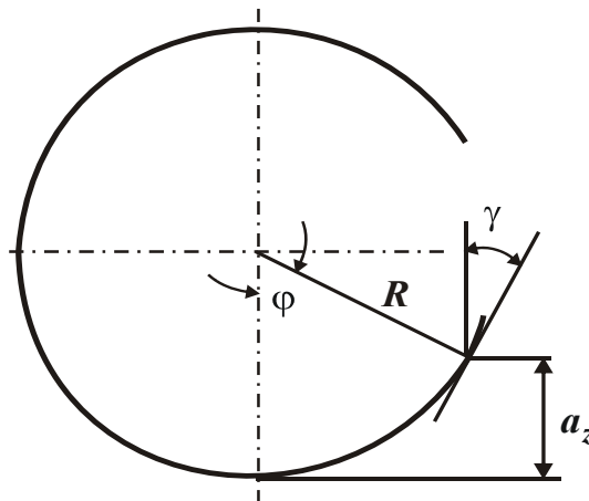
Рис. 1.15. Расчетная схема параметров стружкообразования при микрорезании
