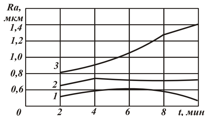
Рис. 3.30. Зависимость параметра шероховатости R_a от времени обработки t :
