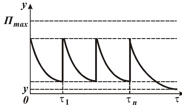
Рис. 3.16. Общий вид зависимости величины y от времени обработки \tau при плоском шлифовании с поперечной подачей
