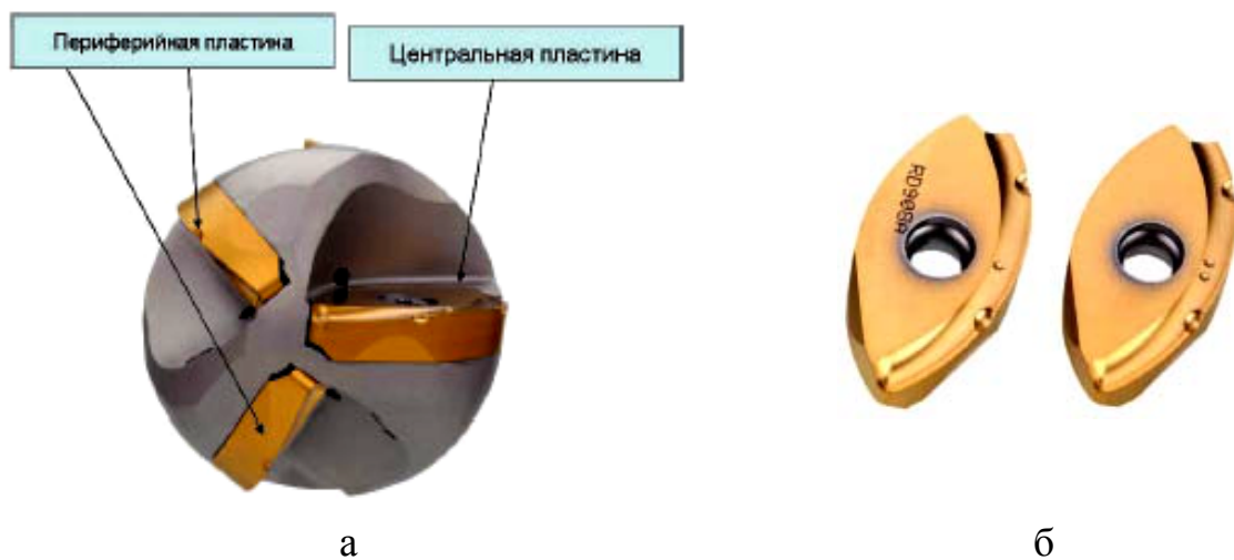
Рис. 6.51. Фреза TRIOBALL с тремя эффективными пластинами (а) и пластина серии 3FBC-M (центральная) и 3FBR-M (периферийная) (б)
