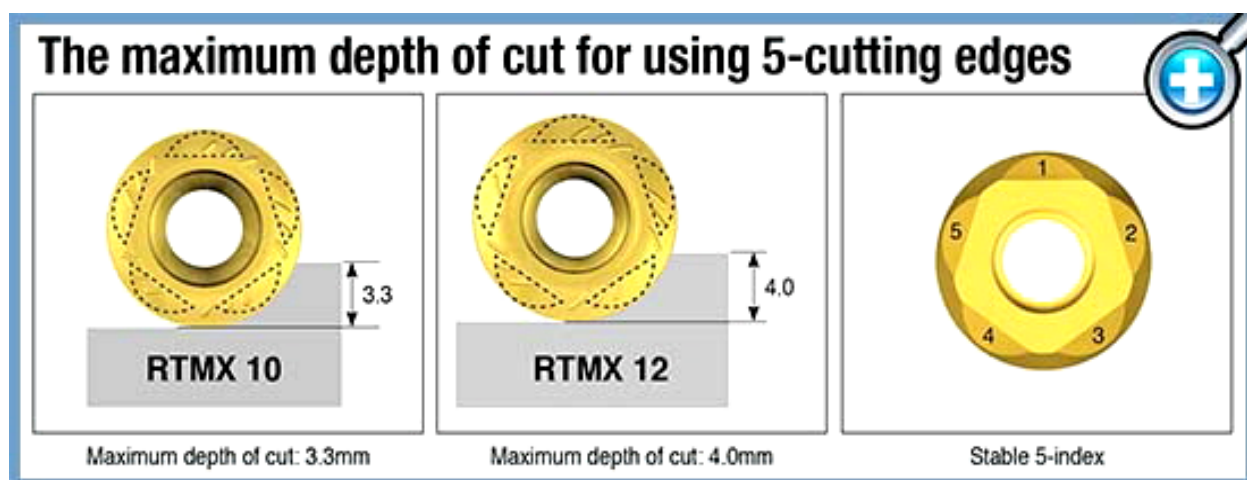
Рис. 6.74. Пластины с тремя стружколомающими геометриями: MM, ML и MLL (а), пластина TaeguTec RTMX с 5 режущими кромками (б)
