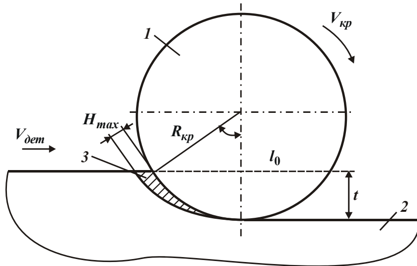
Рис. 5.5. Расчетная схема шлифования:
