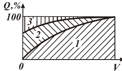
Рис. 4.22. Распределение количества тепла Q , уходящего в стружку (1), заготовку (2) и инструмент (3), при изменении скорости резания V
