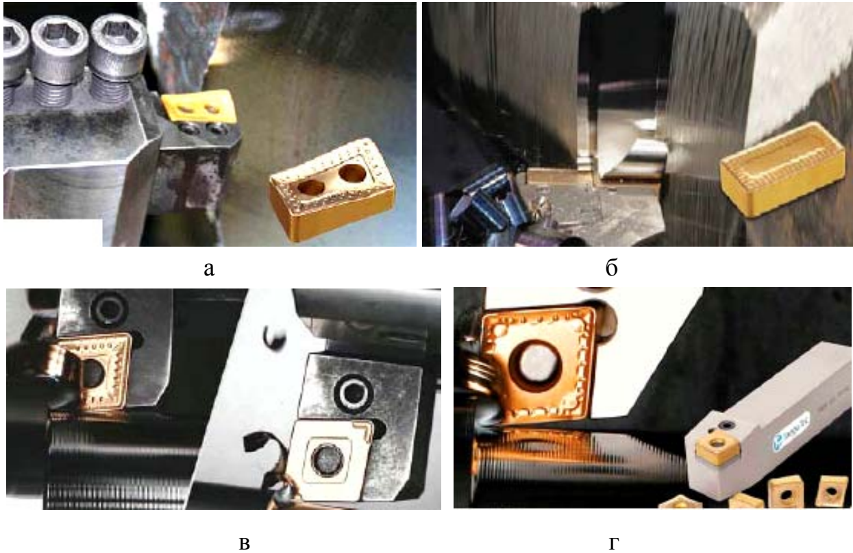
Рис. 6.12. Пластины типа LNMM 40 серии TOP DUTY (а), пластины 50-го типоразмера формы LNMX (б), процесс образования стружки при резании (в), твердосплавные пластины со специальным посадочным местом и стружколомом для получерновой обработки стали (г)
