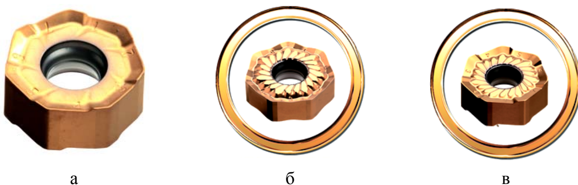
Рис. 6.69. Пластина XNHU 0605 ANN-MM ТТ6080 (а), нейтральная пластина с геометрией ML(б) и с геометрией Wiper для чистовых операций (в)
