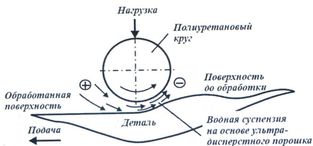
Рис. 1. Схема полирования суспензией на основе ультрадисперсного порошка
