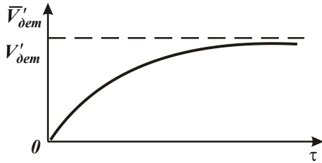
Рис. 2 – Зависимость \bar{V}'_{dem} от \tau
