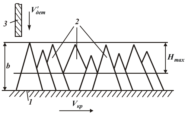
Рис. 1 – Расчетные схемы шлифовании: 1 – связка круга; 2 – режущие зерна; 3 – обрабатываемый образец; 4 – изношенная часть зерна ( V_{кр} – скорость круга, м/с; b – максимальная высота выступания режущих зерен на уровне связки шлифовального круга, м; H_{max} – максимальная толщина среза зернами круга, м)
