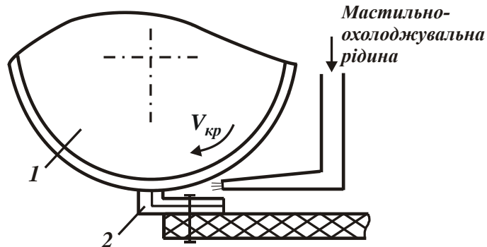
Рисунок 3 – Схема електроерозійної правки алмазного круга (1) з використанням електрода (2), який може утримувати в руках працівника-шліфувальник
