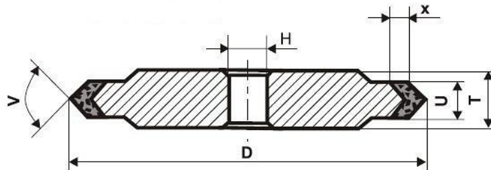
Рисунок 2 – Конусний алмазний круг на металевій зв'язці
