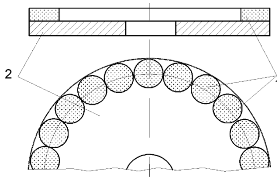
Рисунок 4 – Збірний алмазний круг для торцевого шліфування неметалевих матеріалів підвищеної твердості: 1 – алмазовмісні елементи; 2 - диск
