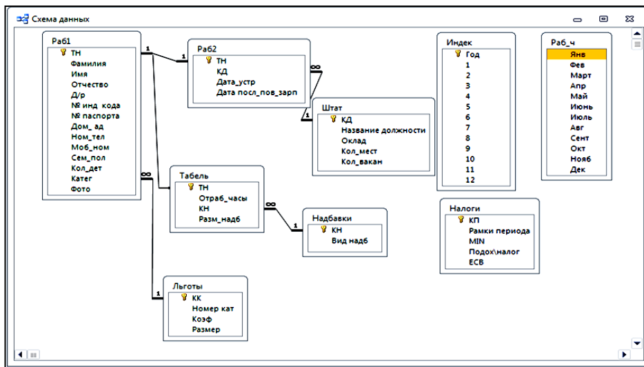
Рис. 1. Схема даних
